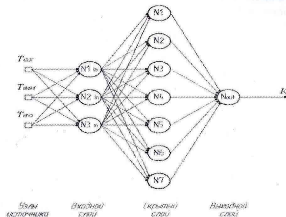
Рис. 4. Структура нейронной сети, трехслойный перцептрон.
