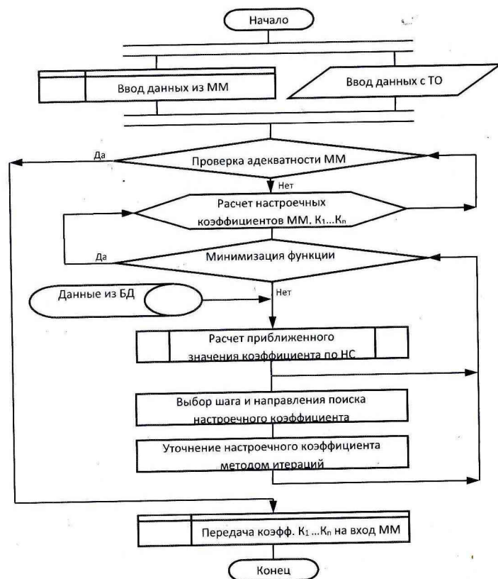
Рис. 3. Обобщенный алгоритм итерационно-нейросетевой идентификации математических моделей ХТП.
