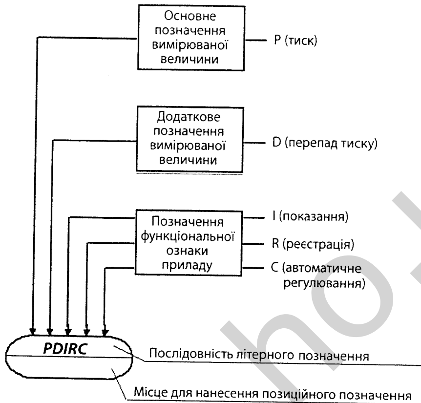
Принцип побудови умовного зображення приладу
